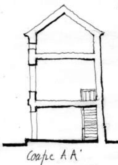
Plan coupé A A'
